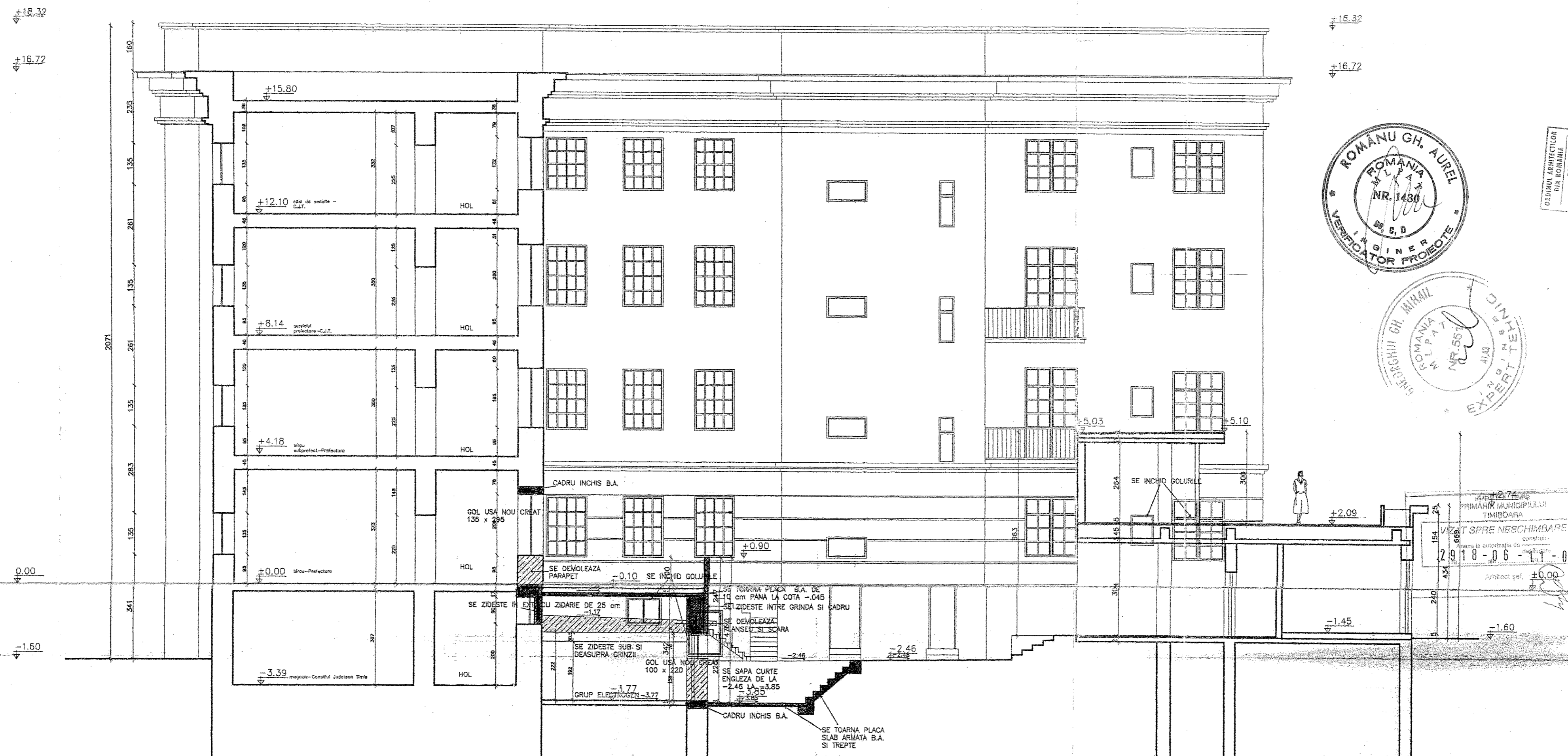
sectiunea A-A'
